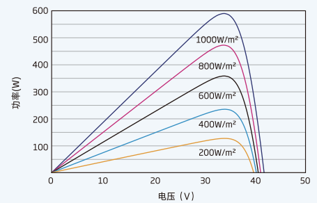
组件的P-V曲线 (595W)
