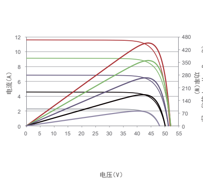
电流电压及功率电压曲线(460W)
